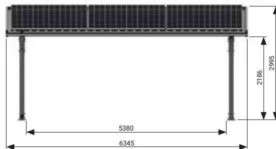
Pogled spredaj - dvojni nadstrešek
