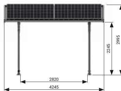
Pogled spredaj - enojni nadstrešek
